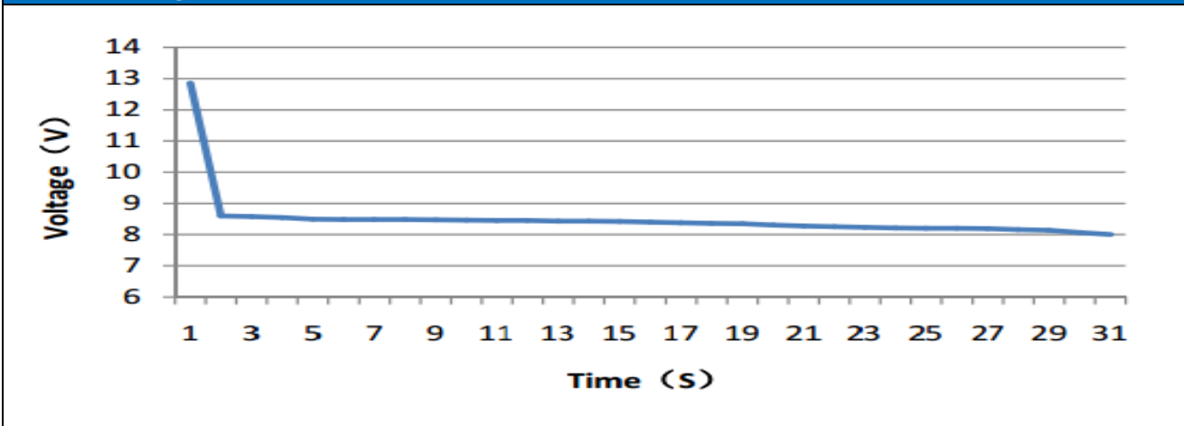
Cold Cranking Test Graph (-18°C, 800CCA)
